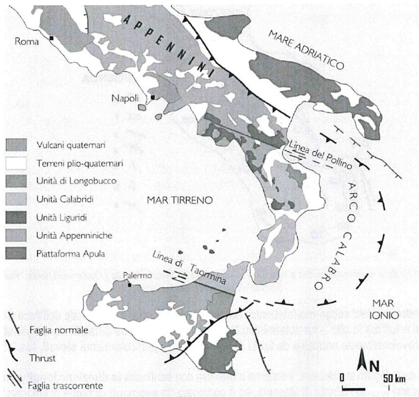
Figura 11. Schema geologico-strutturale semplificato del sistema Appennino meridionale-Arco Calabro (fonte: "Piano Soccorso Rischio Sismico" di Regione Calabria, 2018)
